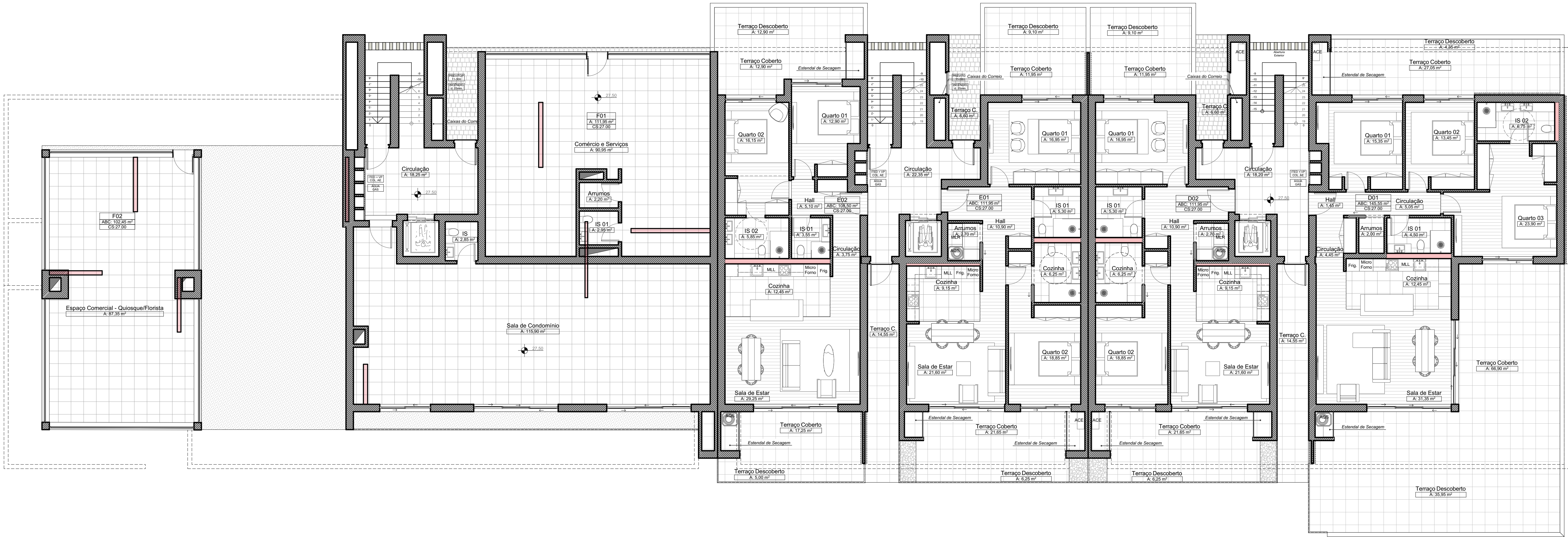
PLANTA DO RÉS-DO-CHÃO - B01
