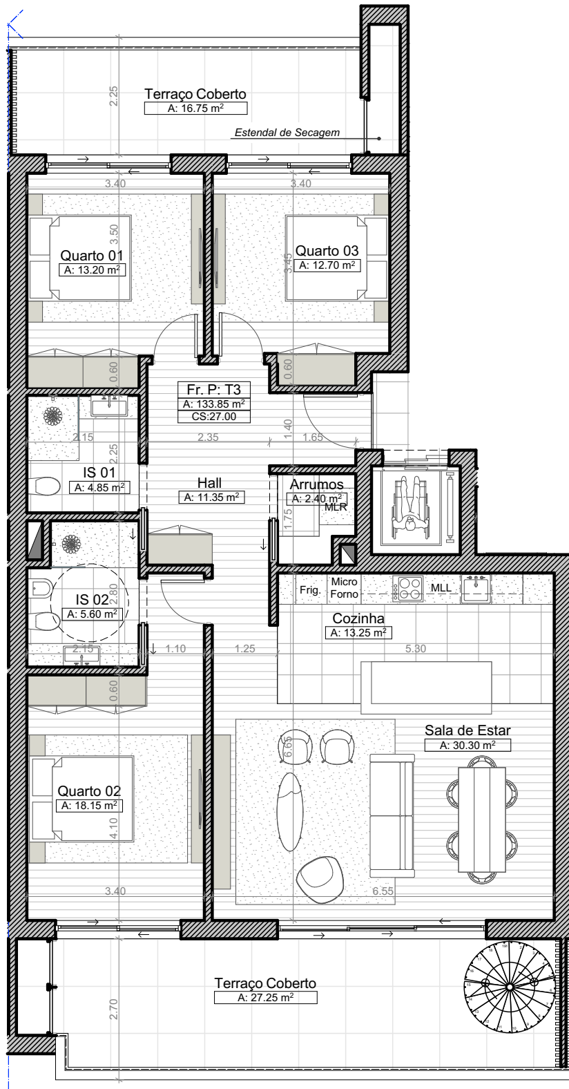
Planta do Apartamento do 2º Andar Esc 1:100
