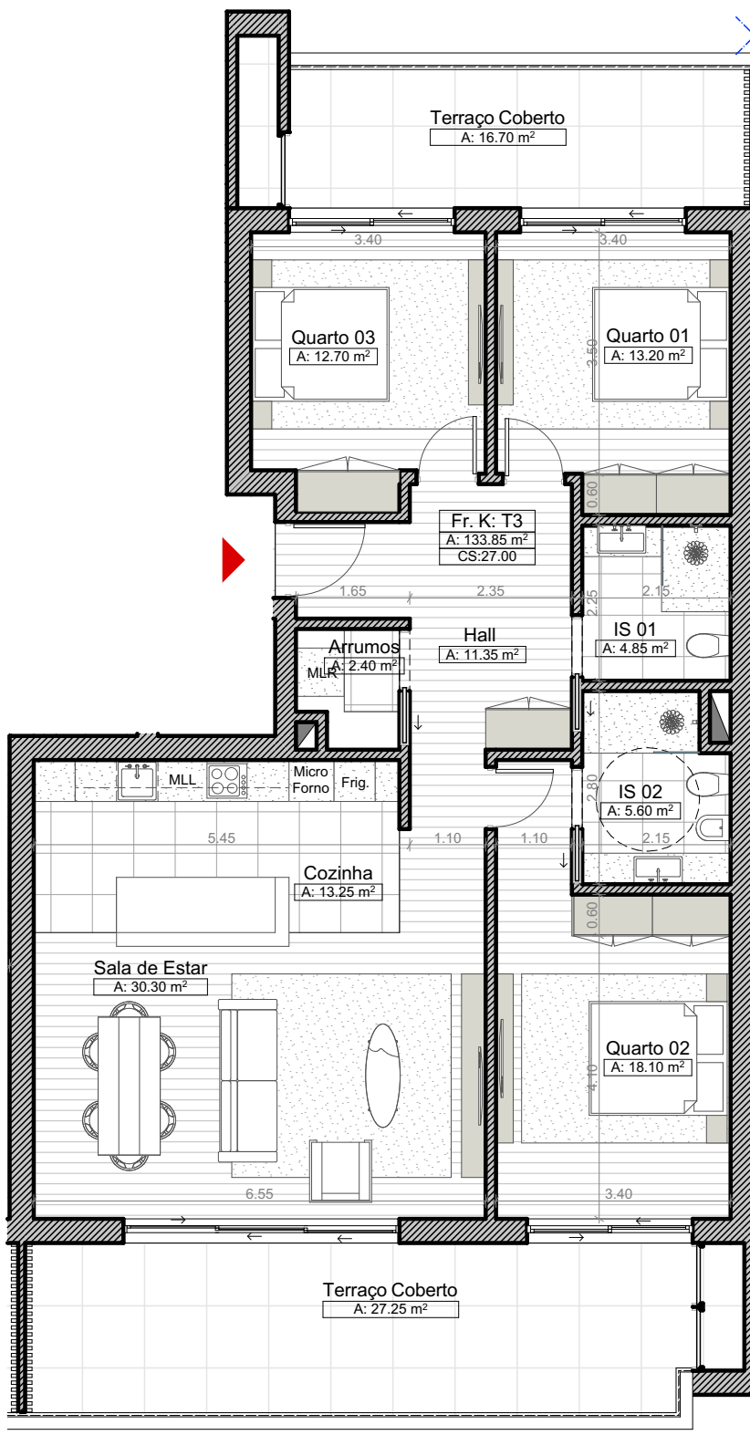
Planta do Apartamento do 1º Andar Esc 1:100
