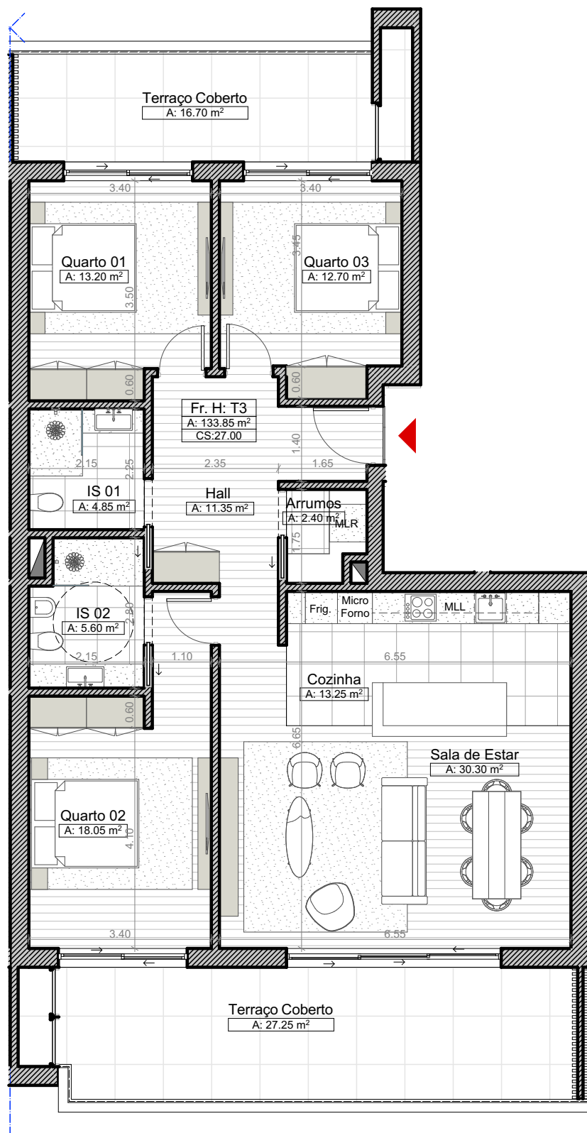
Planta do Apartamento do 1º Andar Esc 1:100
