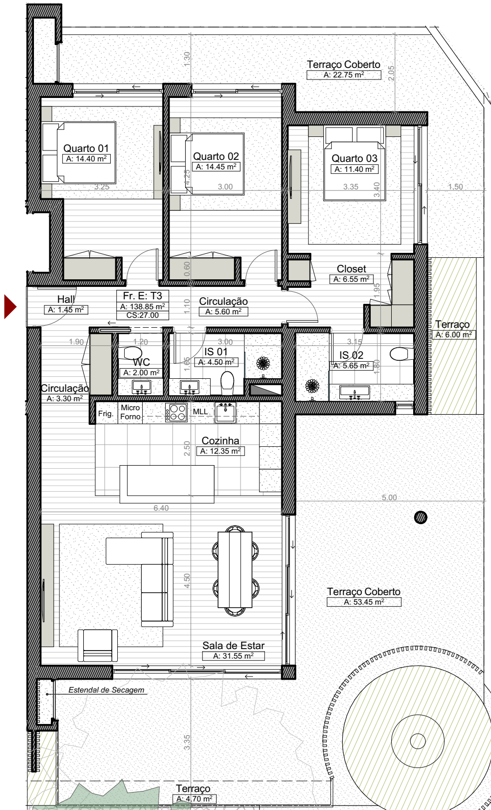
Planta do Apartamento do rés-do-chão Esc 1:100
