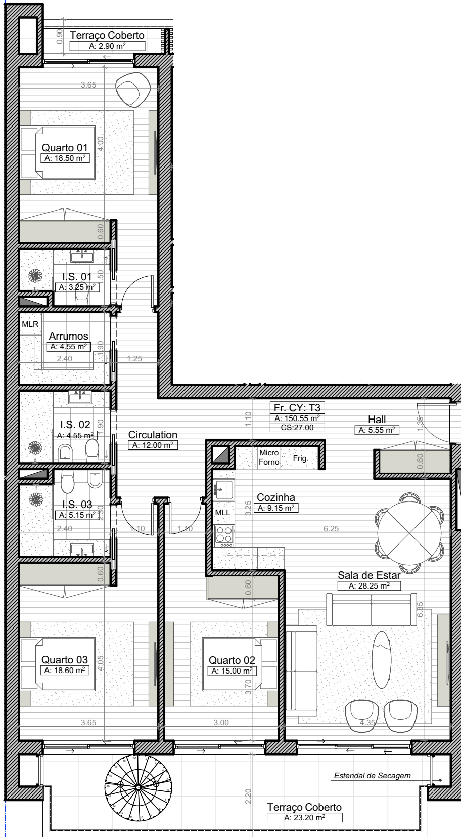
Planta do Apartamento do 2º Andar Esc 1:100
