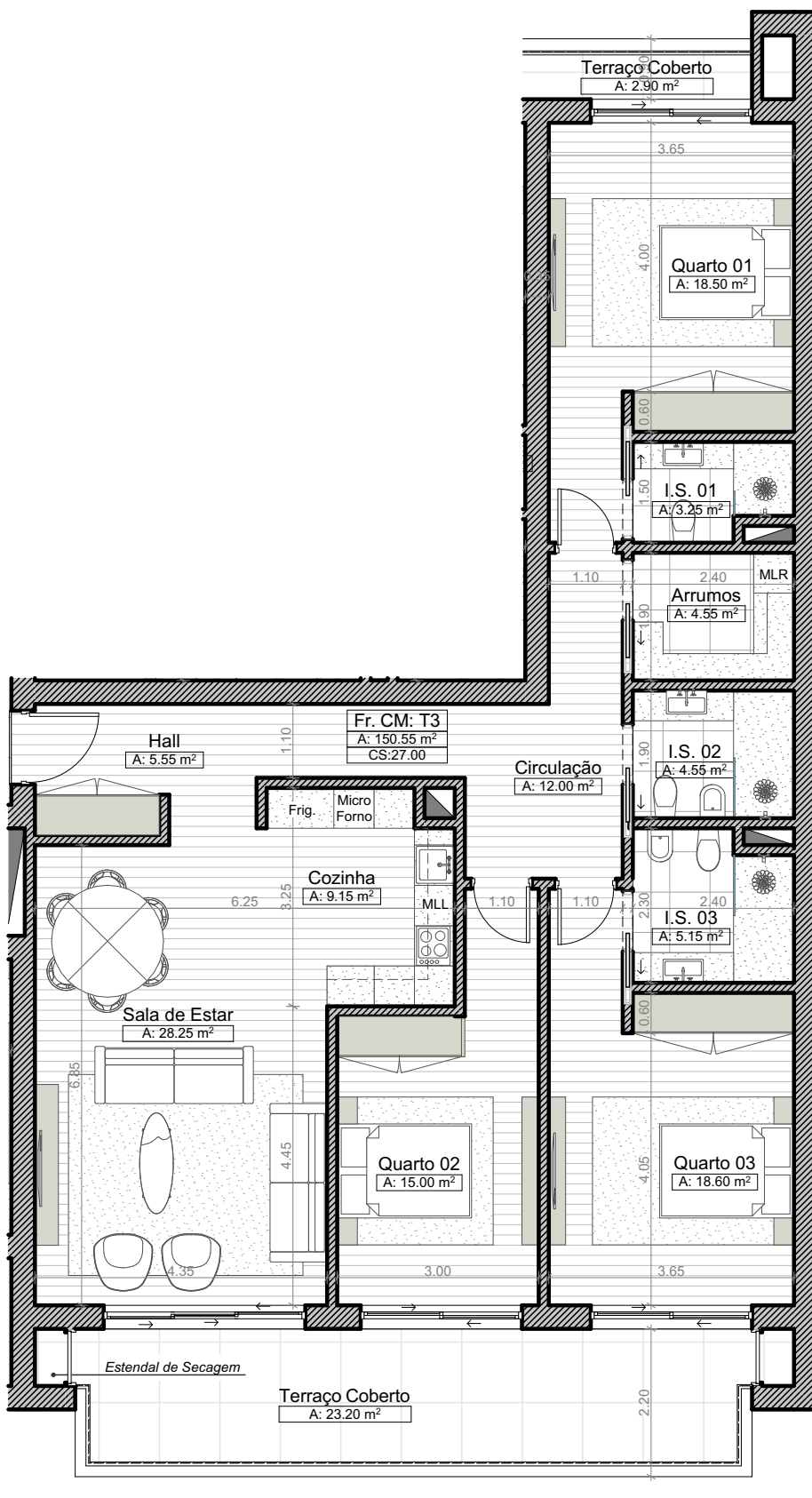
Planta do Apartamento do 1º Andar Esc 1:100
