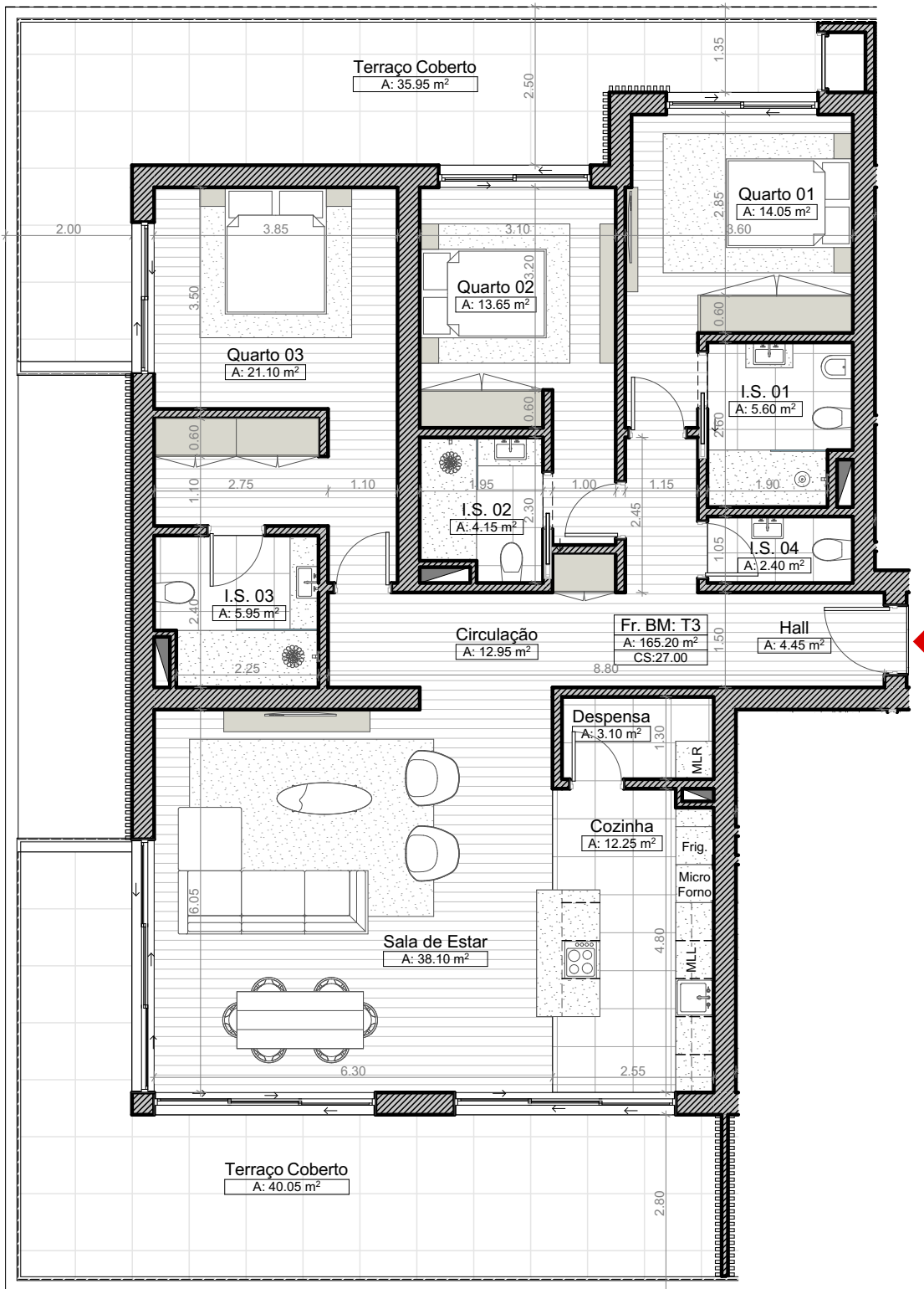
Planta do Apartamento do 1º Andar Esc 1:100
