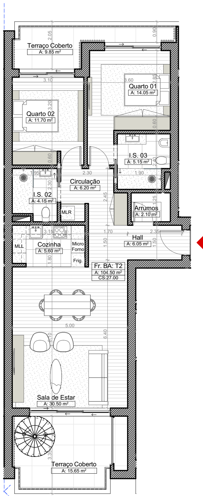
Planta do Apartamento do 2º Andar Esc 1:100
