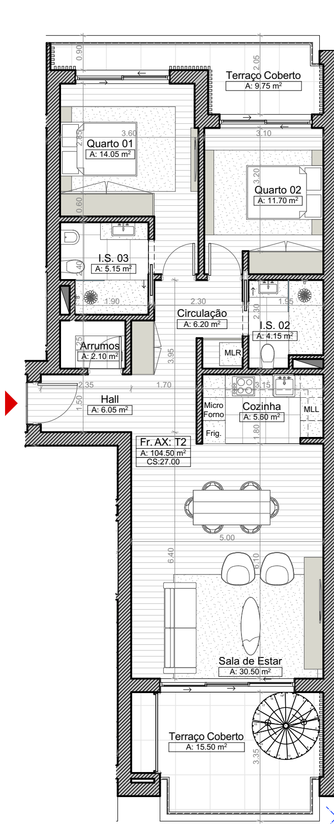
Planta do Apartamento do 2º Andar Esc 1:100
