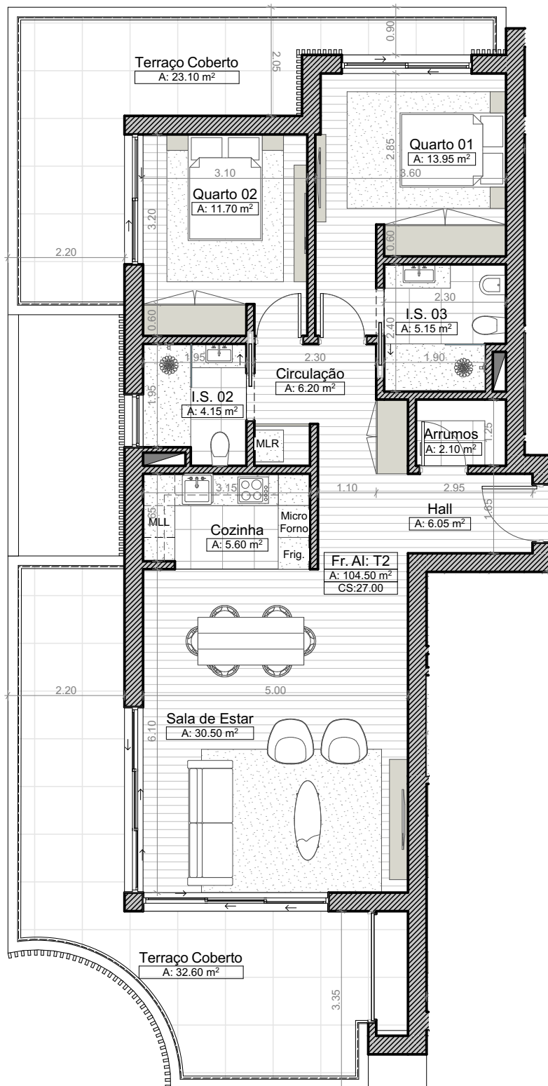
Planta do Apartamento do 1º Andar Esc 1:100
