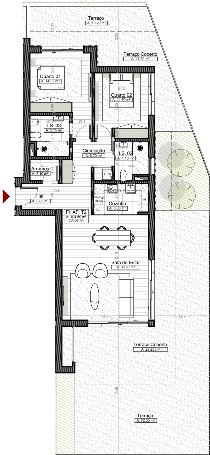
Planta do Apartamento do rés-do-chão Esc 1:125
